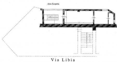
Pianta Piano Primo (H = 2,75 mt.)
