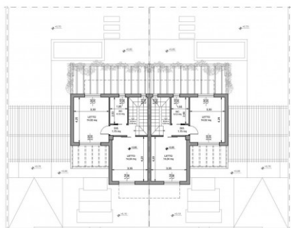
Abitazione Bifamiliare Pianta Piano Primo
