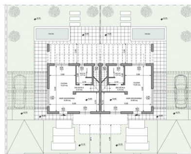
Abitazione Bifamiliare Pianta Piano Terra
